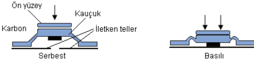
Şekil 78. Kauçuk yapıya sahip anahtarın çalışma prensibi
