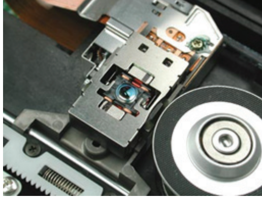
Şekil 62. Optik yazıcı ve lazer ışık kaynağı(howstuffworks.com)
