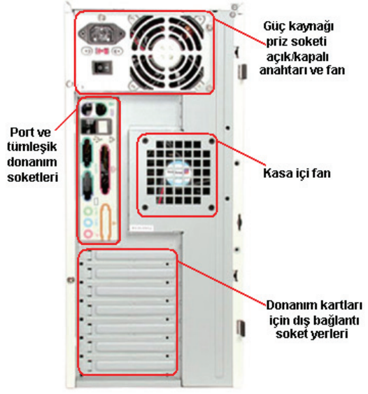
Şekil 113. I. kasanın içyapısı, II. kasanın ön yüzü, III. kasanın arka yüzü
