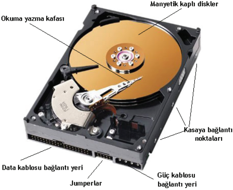
Şekil 35. Sabit diskin iç yapısı ve temel bileşenleri
