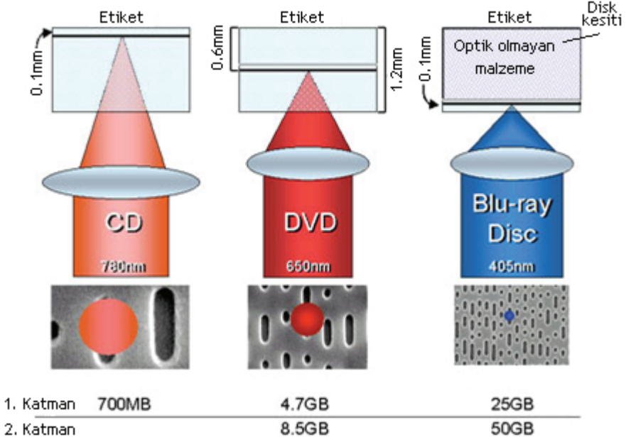
Şekil 57. Disk yapıları(www.pioneerelectronics.com)
