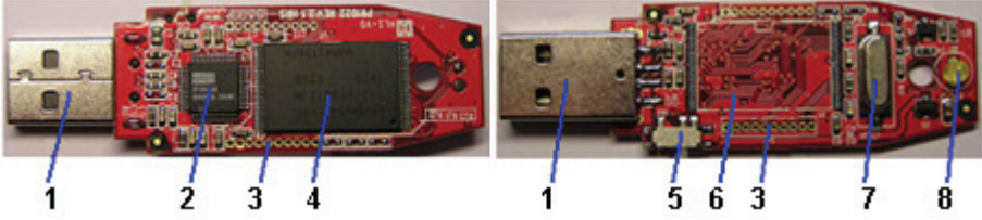
Şekil 100. Flash bellek iç yapısı ve bileşenleri
