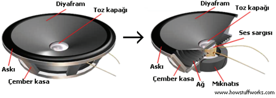
Şekil 96. Hoparlör içyapısı
