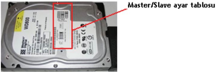
Şekil 42. Master slave ayar tablosunun disk üzerindeki yerleşimi
