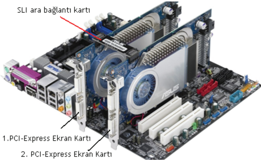
Şekil 18. İki PCI-Express ekran kartının anakarta bağlanmış şekli
