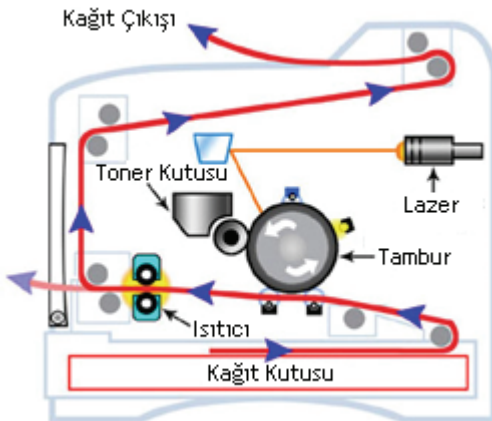
Şekil 69. Lazer yazıcı içyapısı (OKI Inc)
