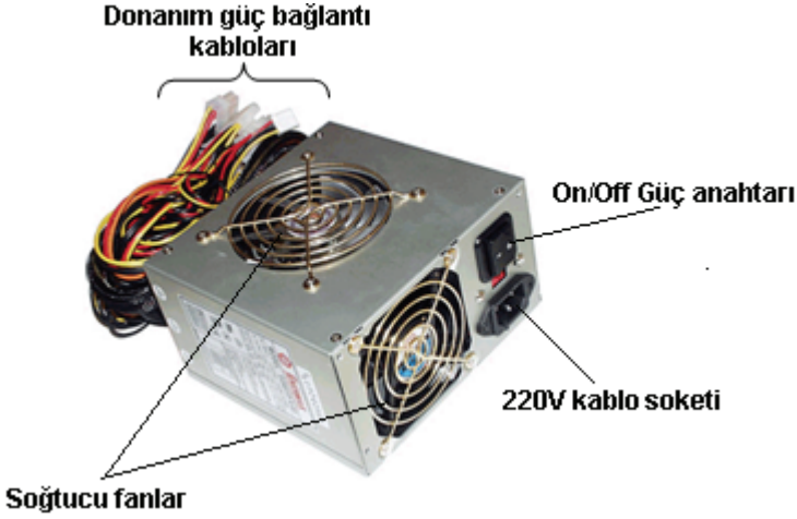
Şekil 114. Güç Kaynağı ve bileşenleri
