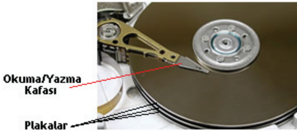
Şekil 37. Plakaların disk üzerindeki yerleşimi
