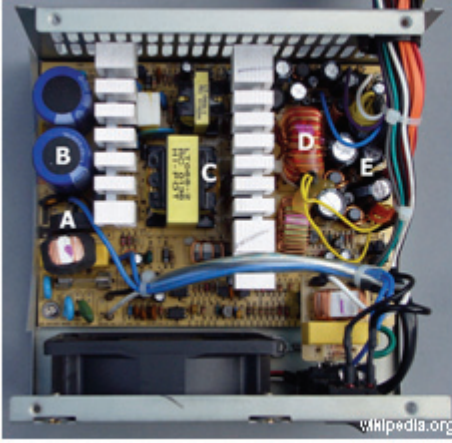
Şekil 116. Güç kaynağının içyapısı ve elektronik parçaları
