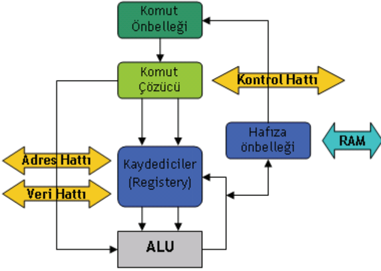
Şekil 26. İşlemcinin temel bileşenleri ve çalışma şekli
