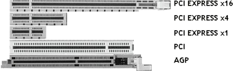
Şekil 19. Çeşitli veriyolu slot yapıları
