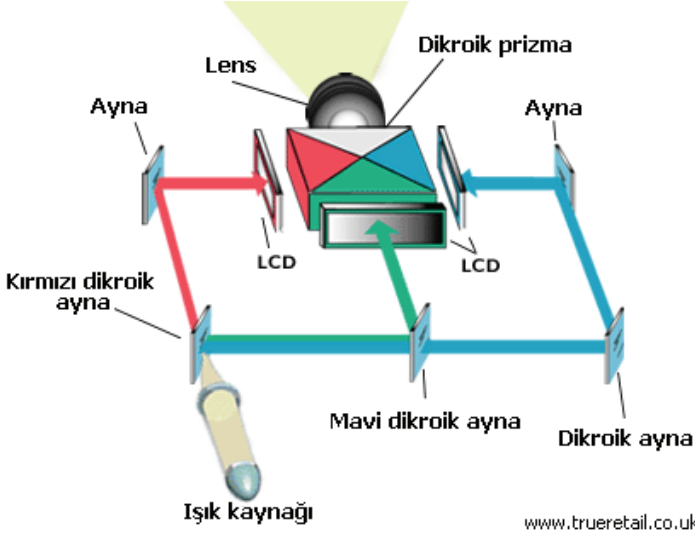
Şekil 90. LCD projeksiyon içyapısı
