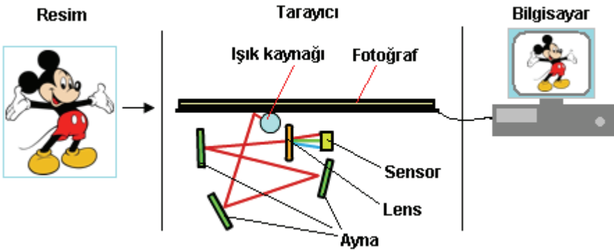
Şekil 118. Tarayıcı bileşenleri
